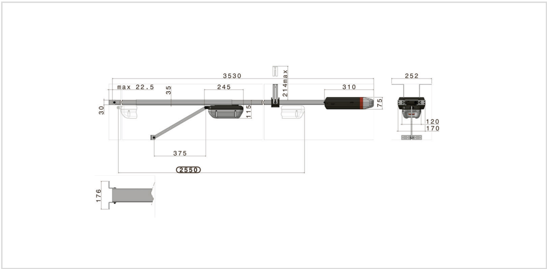
Esempio di motore Sommer Duo Vision 650
